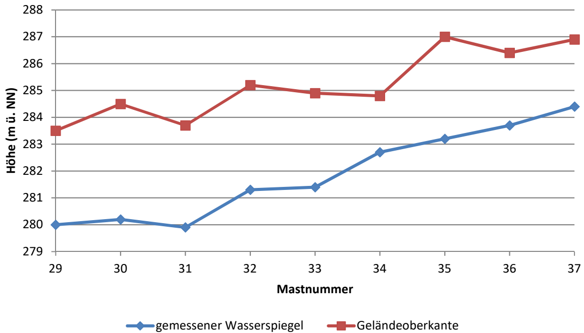
Abbildung 4: Maststandorte 29 bis 37 in Bezug auf den gemessenen Wasserspiegel und Topographie von NW nach SE
